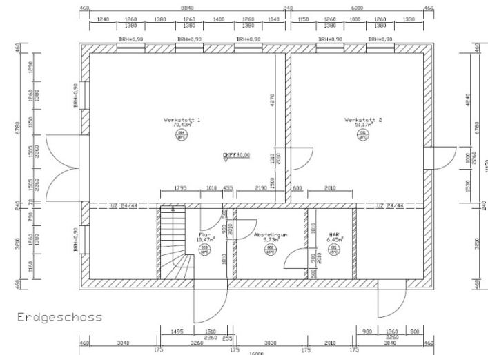
Grundriss Erdgeschoss
